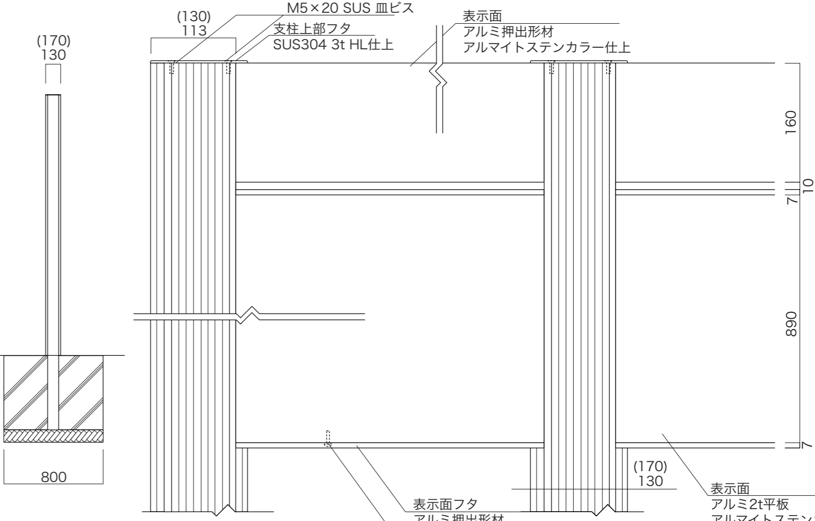
【側面図】
