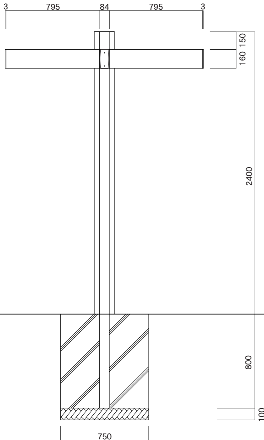
【正面図】
