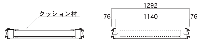
【上面図】
