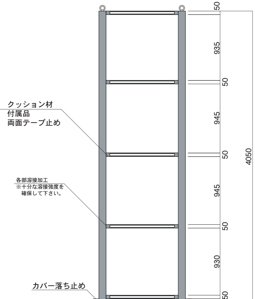
【断面図】
