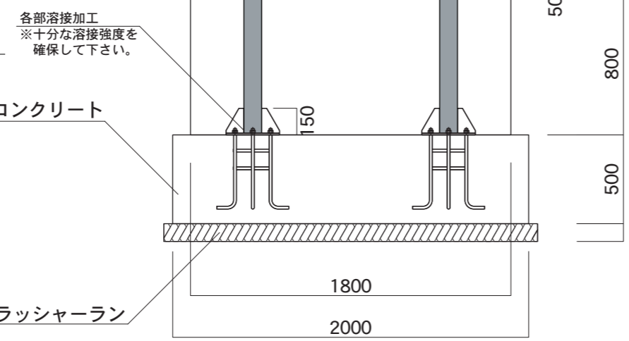
【内部鉄骨正面図】
