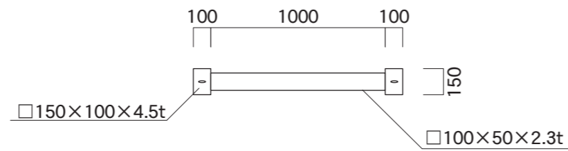
【断面図】
