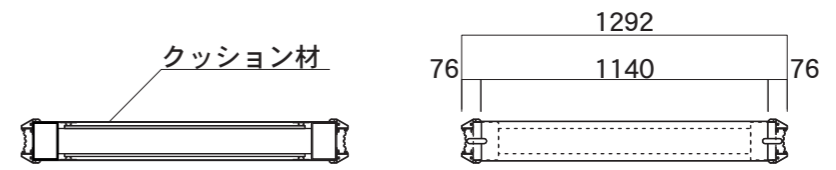
【上面図】
